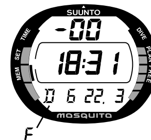
Рис. 5.3. Дневник погружений, Вариант 1.
