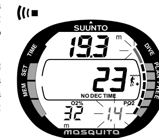
Рис. 3.23 Парциальное давление кислорода и диаграмма OLF. При достижении диаграммы OLF 80% подаются звуковой сигнал и последний сегмент диаграммы начинает мигать. Когда OLF достигает 100%, все сегменты начинают мигать. Если величина OTU больше CNS, то мигает нижний сегмент.
