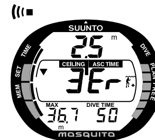
Рис. 3.20 Декомпрессионное погружение, глубина меньше глубины потолка. Обратите внимание на направленную вниз стрелку, предупредительную Eg и звуковой сигнал. Вы должны немедленно (в течение 3 минут) погрузиться ниже потолка.
