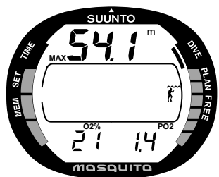
Рис. 3.21 Дисплей NITROX. Максимальная глубина погружения при текущих параметрах смеси (21% O 2 и 1.4 бар. PO 2 ) - 54.1 м.
