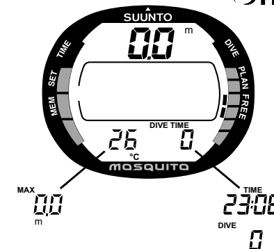
Рис. 3.5. Активация. Шаг IV. Режим FREE/GAUGE. Текущая глубина и время погружения равны нулю. Нажатием +/- отображается максимальная глубина, текущее время или номер погружения.
