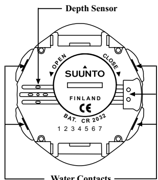
Рис. 2.2. Водоактивируемый контакт и датчик глубины.
