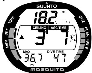
Рис. 3.17 Декомпрессионное погружение, глубина больше глубины пола. Стрелка, направленная вверх, мигающая надпись ASC TIME и звуковой сигнал напоминают о необходимости всплытия. Минимальное время всплытия с учетом остановки безопасности - 7 минут. Глубина потолка 3 метра.
