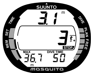
Рис. 3.12. Трехминутная рекомендуемая остановка безопасности.
