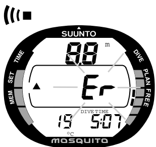
Рис. 3.32. Дисплей после превышения лимита в 5 мин. Мигающая надпись Er и стрелка вверх.
