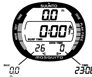
Рис. 3.4. Активация. Шаг III. Режим Поверхности (AIR). Глубина и время погружения равны нулю. Нажатием +/- отображается максимальная глубина и текущее время.
