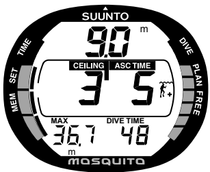
Рис. 3.18 Декомпрессионное погружение, Вы находитесь над полом. Стрелка, направленная вверх, исчезла, а надпись ASC TIME не мигает. Началось рассыхание тканей организма от азота.
