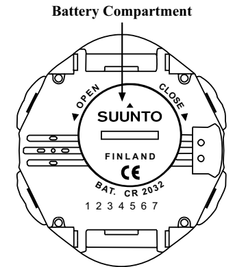
Рис. 6.1. Отсек источника питания.
