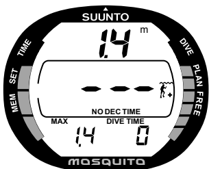
Рис. 3.10. Погружение только что началось. Доступное время бездекомпрессионного погружения более 199 мин.
