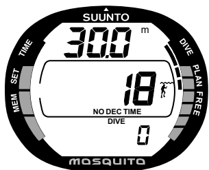
Рис. 3.9. Планирование. Допустимое время бездекомпрессионного погружения в режиме PO/AO на глубине 30 м - 18 минут.
