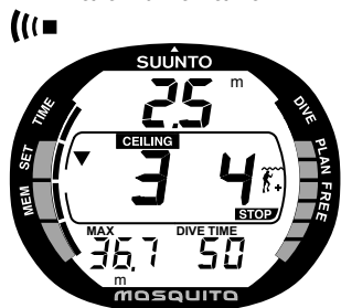
Рис. 3.13. Обязательная остановка безопасности. Вам рекомендуется выполнить обязательную остановку безопасности в диапазоне глубин между полом и потолком.
