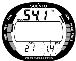
Рис. 4.9. Установка процентного содержания O 2 в ДГС и величины парциального давления кислорода.
