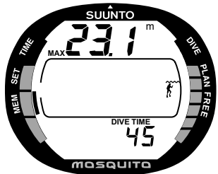
Рис. 5.4. Дневник погружений, Вариант II. Основные данные о погружении.
