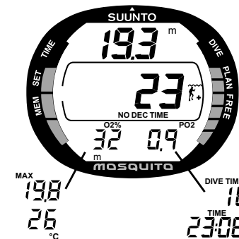
Рис. 3.22 Погружение в режиме EAN. Значение O 2 % - 32%.
