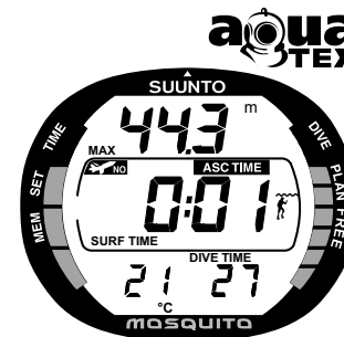
Рис. 3.26 Режим Поверхности после пропуска декомпрессионной остановки. Надпись ASC TIME означает пропуск декомпрессионной остановки. Вы не должны совершать погружений в течение 48 ч.
