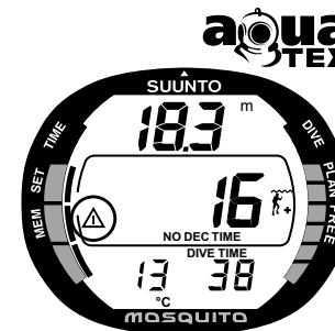
Рис. 3.7. Внесение специальных пометок в память декомпрессиметра. С помощью кнопки S Вы можете сделать специальную пометку в памяти профилей погружений (появится значок «Обратите внимание!»).
