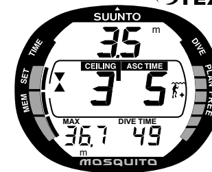
Рис. 3.19 Декомпрессионное погружение, глубина зоны потолка. Две стрелки, направленные друг на друга, указывают, что Вы в зоне потолка (глубина 3.5 м.). Минимальное время всплытия 5 минут.
