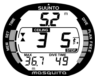
Рис. 3.13. Обязательная остановка безопасности. Вам рекомендуется выполнить обязательную остановку безопасности в диапазоне глубин между полом и потолком.
