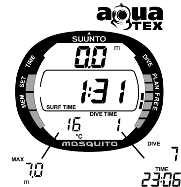
Рис. 3.33. Внешний вид дисплея после фридайвинга. В центре дисплея отображается время нахождения на поверхности.
