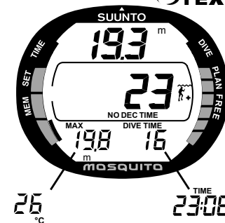
Рис. 3.11 Режим Погружения. Текущая глубина 19.3 м, оставшееся время бездекомпрессионного погружения в режиме A0/P1 - 23 минуты. Макс. глубина погружения 19.8 м., время погружения 16 мин. и температура воды 18 °C. При нажатии на кнопки +/- будет отображаться температура воды и текущее время.
