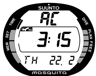
Рис. 2.3. При замыкании водоактивируемого контакта на дисплее появляется надпись AC.
