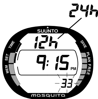
Рис. 4.3. Включен режим настройки времени. Значение секунд начинает мигать.
